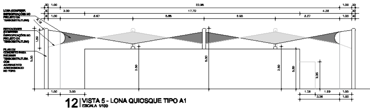
Imagem 12 – Vista lateral da estrutura tensionada acima das edificações (blocos tipo A). Fonte: COPROJ-SEINF.
