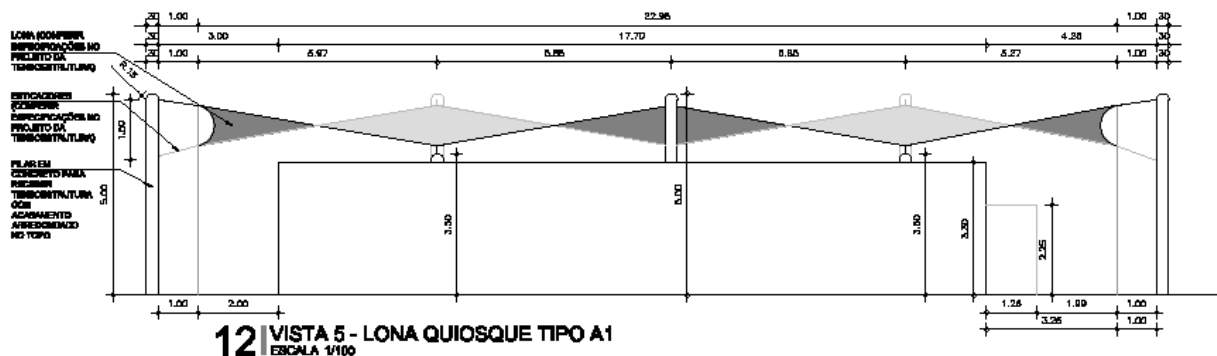
Imagem 03 – Vista lateral da estrutura tensionada acima das edificações (blocos tipo A).
